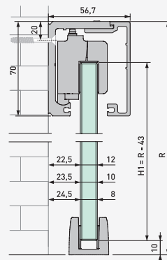
Dubbelvleugelige installatie zonder vast zijpaneel
