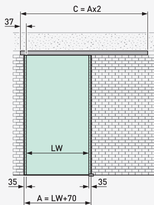
Enkelvleugelige installatie zonder vast zijpaneel
