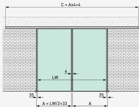
Dubbelvleugelige installatie zonder vast zijpaneel
