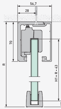
Enkelvleugelige installatie zonder vast zijpaneel
